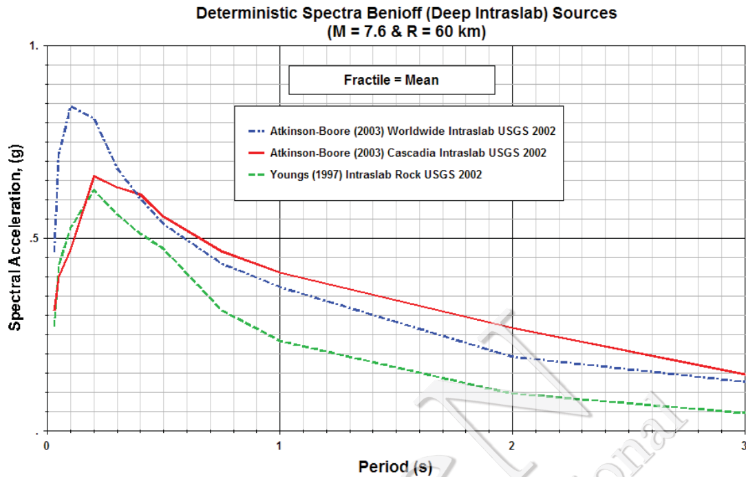
Gambar V-15. Respon Spektra untuk sumber gempa Benioff ( Deep Background / intralab ) (Asrurifak, 2010)
