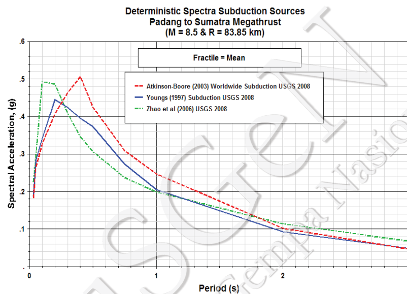
Gambar V-13. Grafik Respon Spektra untuk sumber gempa Subduksi ( interface ) (Asrurifak, 2010)
