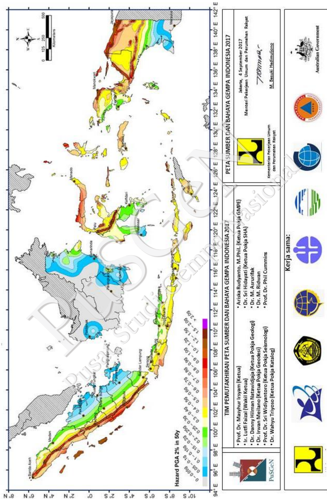
D10: Peta percepatan puncak di batuan dasar (SB) untuk probabilitas terlampaui 2% dalam 50 tahun
