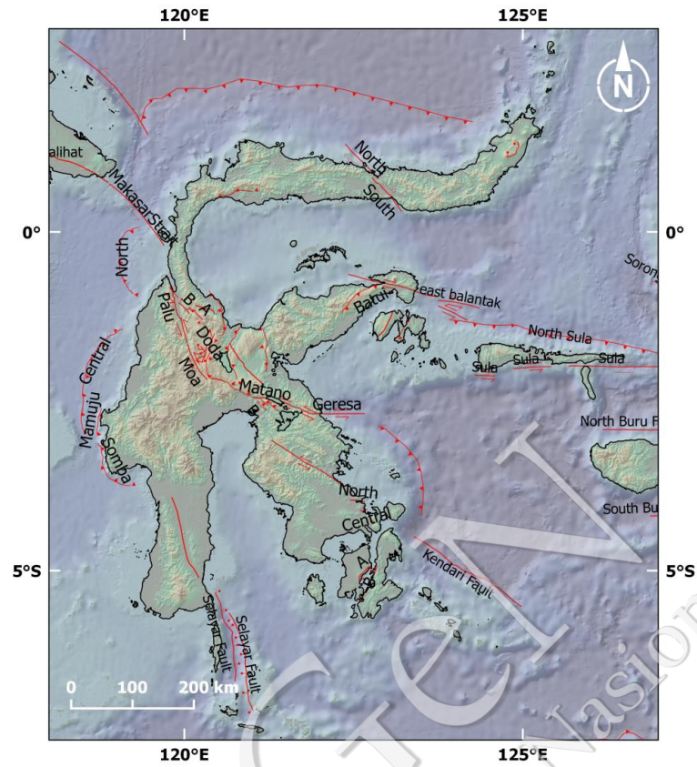
Gambar II-19. Peta Sesar Aktif di Pulau Sulawesi Yang Terangkum Dalam Peta Gempa Nasional 2017
