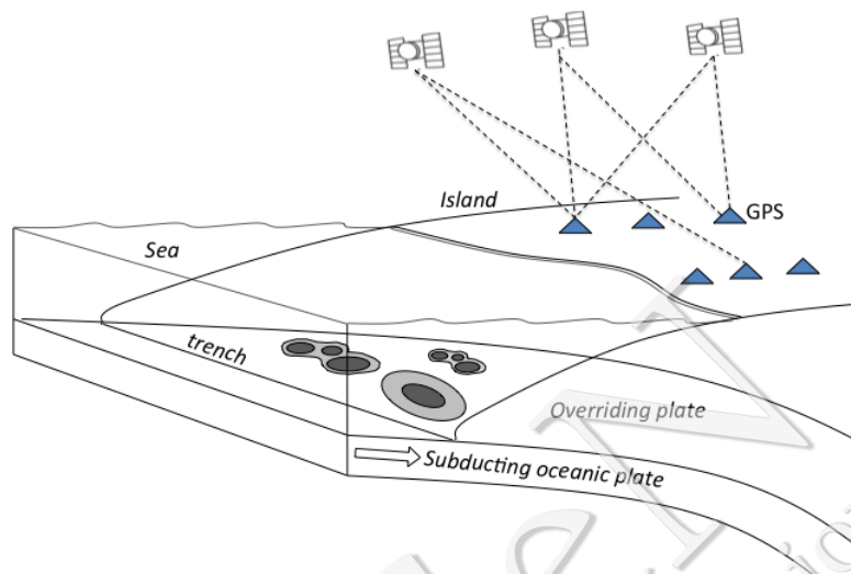
Gambar IV-2. Ilustrasi Pemanfaatan Data GPS untuk Analisis Tektonik. (Hanifa, 2014, yang digambar dengan modifikasi dari Wang dkk., 2012)
