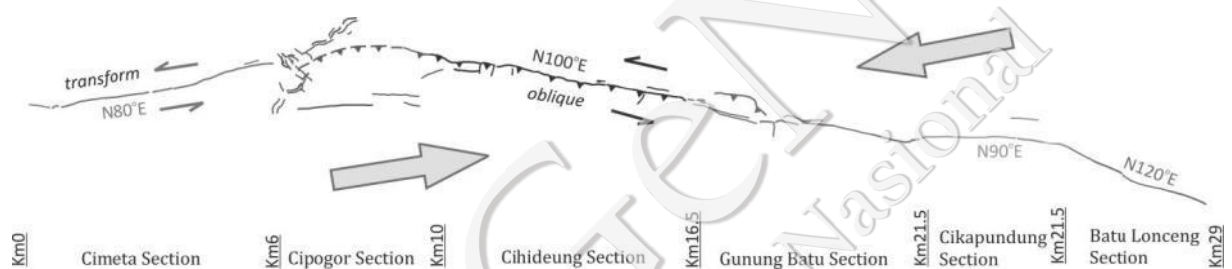
Gambar II-15. Kinematika Sesar Lembang dan Pembagiannya menurut Daryono (2016)
