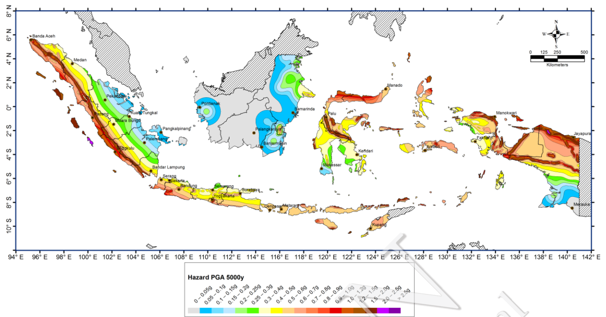
Gambar VI-23. Peta percepatan puncak di batuan dasar (SB) untuk probabilitas terlampaui 2% dalam 100 tahun
