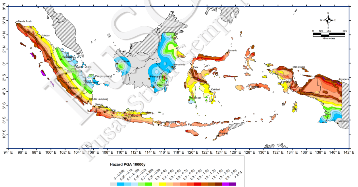
Gambar VI-24. Peta percepatan puncak di batuan dasar (SB) untuk probabilitas terlampaui 1% dalam 100 tahun
