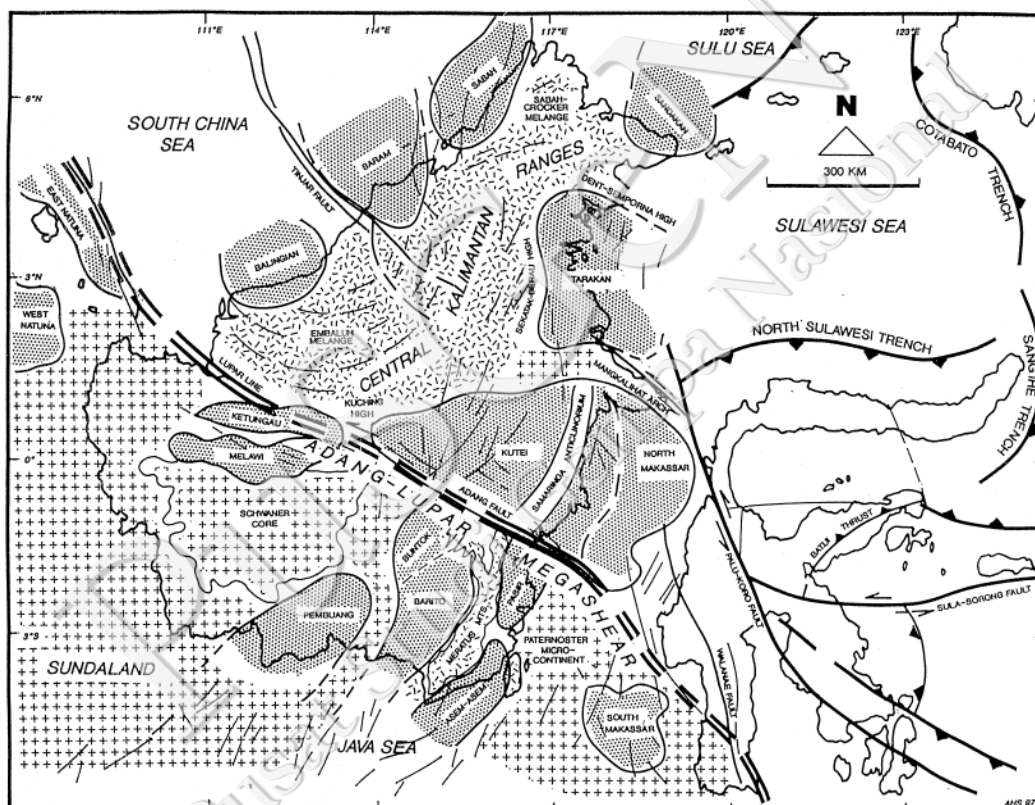
Gambar II-29. Kerangka Tektonik Pulau Kalimantan dan Sekitarnya (Satyana dkk., 1999)
