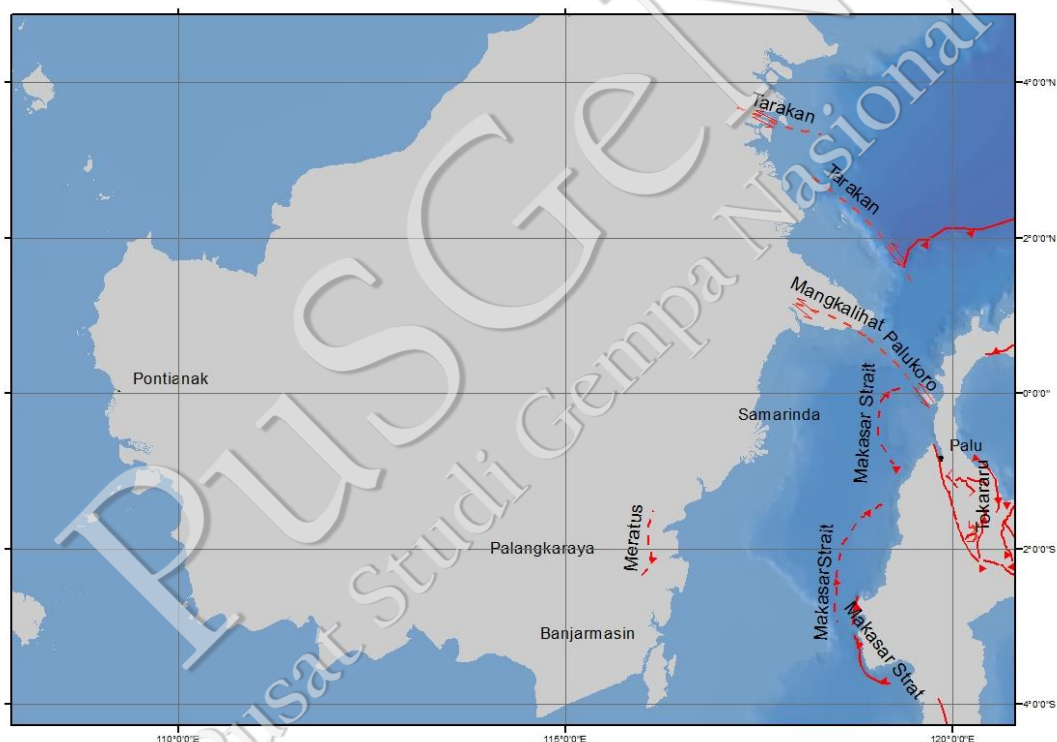
Gambar II-30. Sebaran Sesar Aktif yang Berhasil Diidentifikasi di Kalimantan yang Terangkum dalam Peta Gempa Nasional 2017
