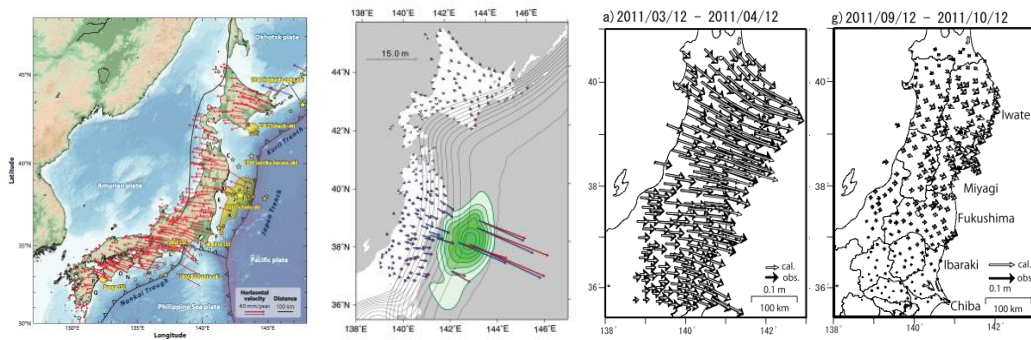
Gambar IV-4. (kiri) Fase interseismic (sebelum) pada September 2007 – Februari 2011 (Nishimura dkk., 2014); arah kecepatan menjauhi trench /searah dengan arah konvergensi lempeng pasifik. (tengah) Fase koseismik (saat gempa) pada Gempa Tohoku Jepang 2011 M9.0 (Hashimoto dkk., 2012); arah deformasi menuju trench . (kanan) Fase postseismik (sesudah gempa); arah deformasi menuju trench dengan magnitude yang lebih kecil dari deformasi koseismik (Ozawa dkk., 2012)
