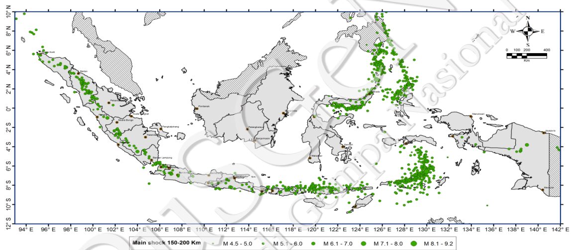
Gambar VI-9. Peta episenter gempa pada kedalaman 150-200 km pada periode 1900-2016 yang digunakan sebagai sumber gempa deep-3 background
