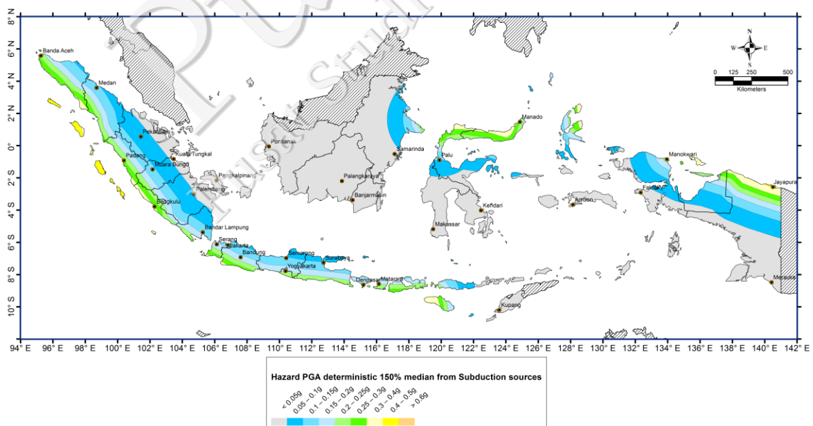
Gambar VI-12. Peta Bahaya Gempa deterministik PGA di batuan dasar akibat sumber gempa subduksi dengan 84 percentile (150% median)
