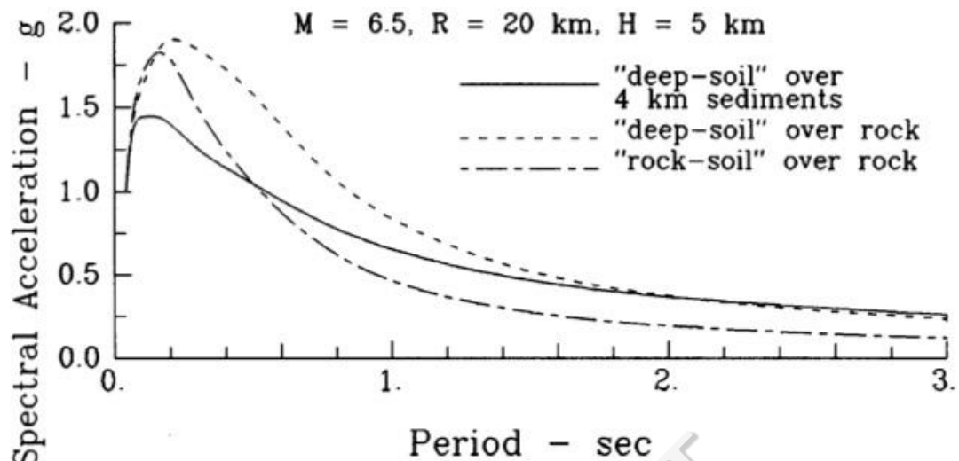
Gambar V-7. Ilustrasi pengaruh jenis tanah terhadap spektral akselerasi suatu gempa (dimodifikasi dari Gupta, 2002)
