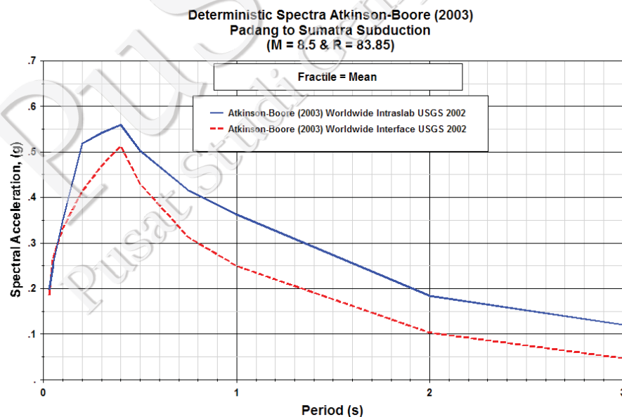
Gambar V-12. Grafik Respon Spektra persamaan GMPE Atkinson-Boore (2003) untuk sumber gempa Deep Background (intraslab) dan Subduksi (interface) (Asrurifak, 2010)
