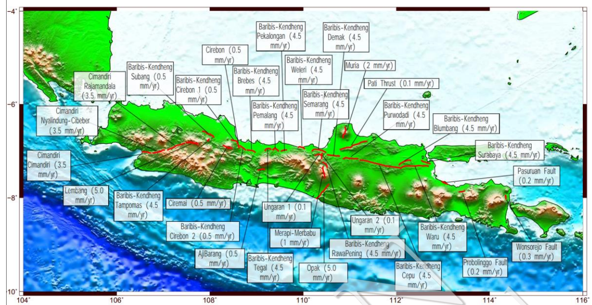
Gambar IV-41. Laju geser segmen-segmen sesar di Jawa
