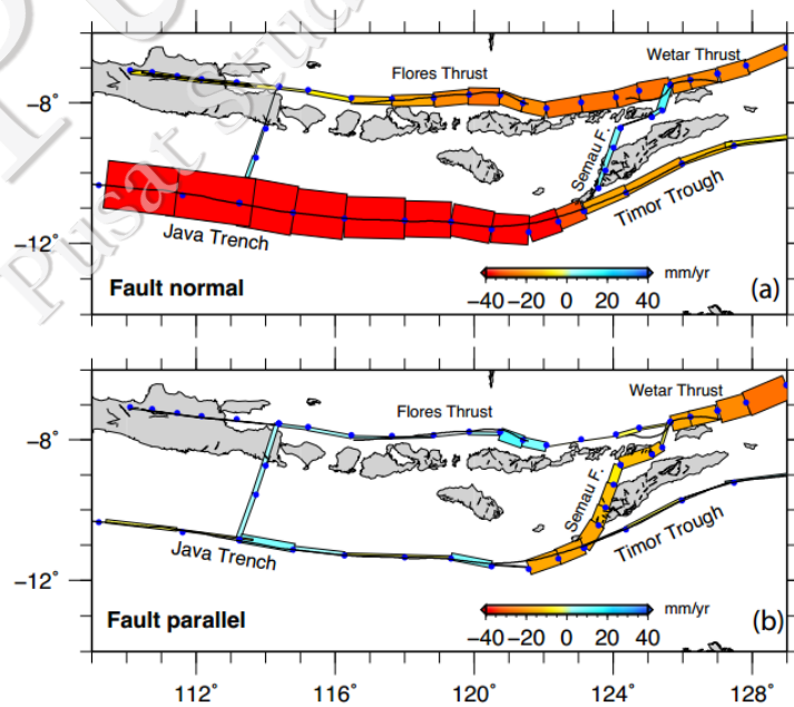
Gambar IV-58. Sliprate Jawa Bagian Timur – NTT (Koulali dkk., 2016a)
