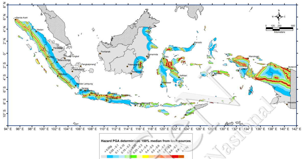
Gambar VI-11. Peta Bahaya Gempa deterministik PGA di batuan dasar akibat sumber gempa sesar dangkal dengan 84 percentile (150% median)
