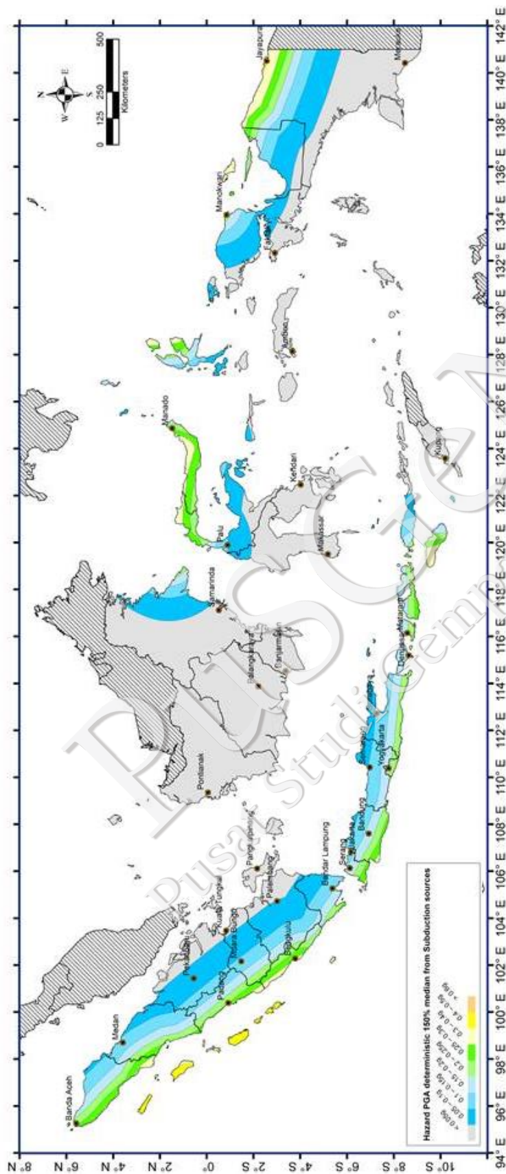
D2: Peta percepatan puncak di batuan dasar (SB) deterministik akibat sumber gempa Subduksi dengan 84-percentile (150% Median)
