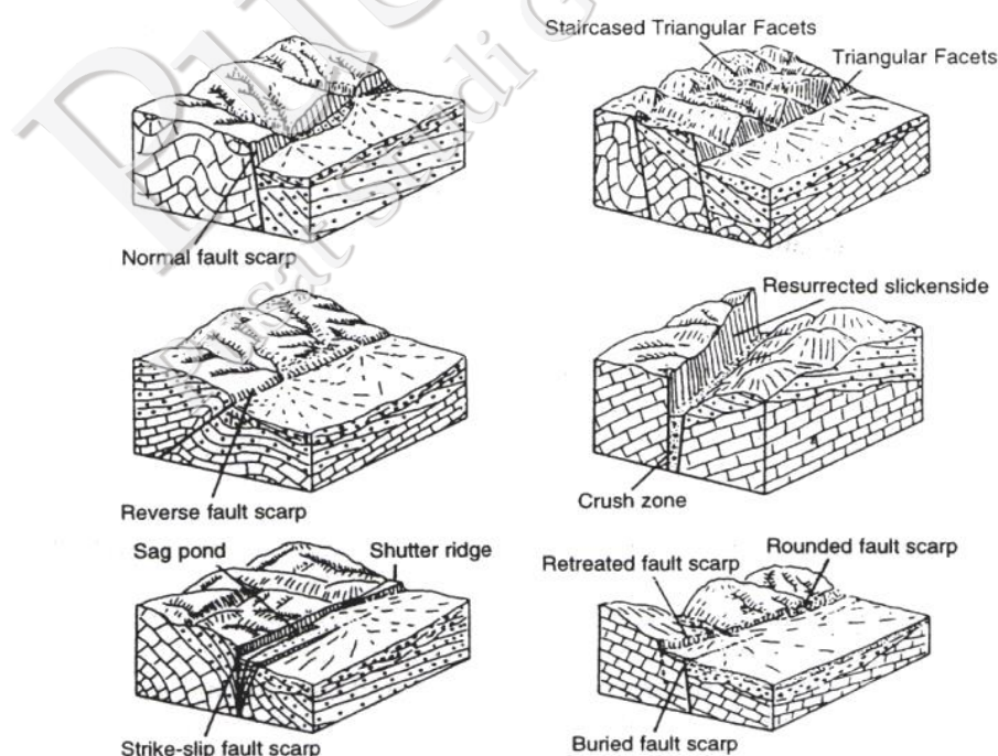
Gambar II-1. Bentuk morfologi yang berhubungan dengan sesar aktif. Bentuk-bentuk tersebut diberi simbol berdasarkan morfologi yang muncul (McCalpin, 1996)
