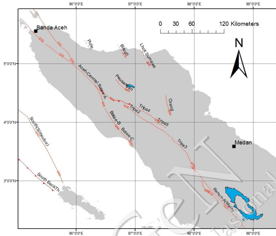
Gambar II-7. Sesar-Sesar Aktif Dan Segmen Yang Ada Di Wilayah Sumatra Bagian Utara Yang Terangkum Dalam Peta Gempa Nasional 2017
