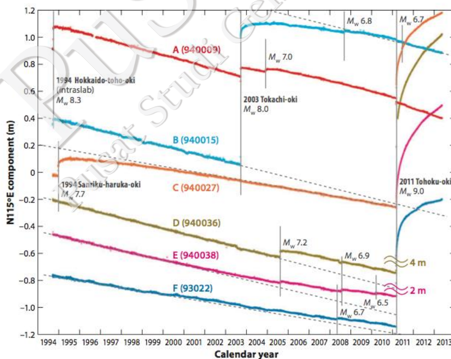
Gambar IV-3. Contoh Data Time Series GPS di Jepang dari tahun 1994 hingga 2013 (Nishimura dkk., 2014). Garis vertikal hitam menunjukkan waktu terjadi gempa. Terlihat pola interseismik (sebelum gempa), offset coseismik (pada waktu terjadi gempa), dan pola postseismik (sesudah gempa)
