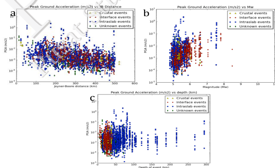
Gambar V-9. Distribusi data yang digunakan dalam perbandingan GMPE pada Tabel V-1. a) berdasarkan jarak Joyner-Boore, b) berdasarkan magnitude, dan c) berdasarkan kedalaman (Ariska, 2013)
