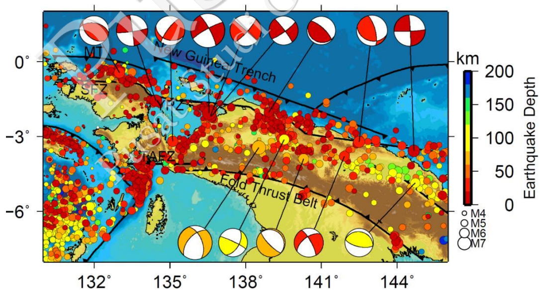
Gambar III-24. Episenter gempa hasil relokasi di zona Papua dan sekitarnya untuk event dengan kedalaman \leq 200 km dan magnitudo \geq 4 . Mekanisme fokus merupakan solusi dari GCMT untuk gempa dengan magnitudo \geq 6 (Shiddiqi, 2015). Singkatan: MT: Manokwari trench , SFZ: zona sesar Sorong, YPZ: zona sesar Yapen, TAFZ: zona sesar Tarera Aiduna. Struktur sesar aktif berdasarkan Sapiie (1998)
