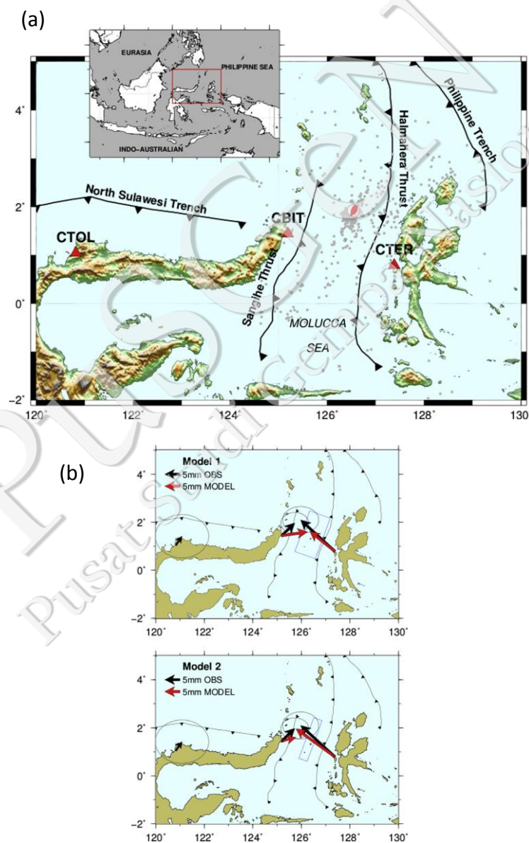
Gambar IV-50. Penelitian terbaru oleh Gunawan dkk., 2016 membuktikan bahwa terjadi splay-fault rupture selama mainshock dari Gempa Maluku 2014 M_w = 7,1 . Pengamatan ini menggunakan data dari dua stasiun GPS di sekitar Laut Maluku
