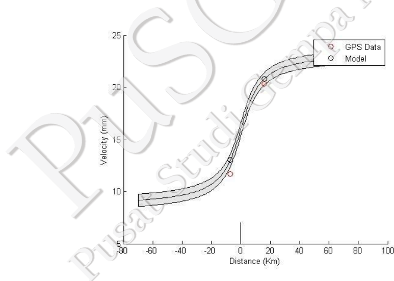
Gambar IV-44. Perhitungan laju geser Sesar Palu-Koro dengan menggunakan metode Simple Screw Dislocation (Savage and Burford, 1973)
