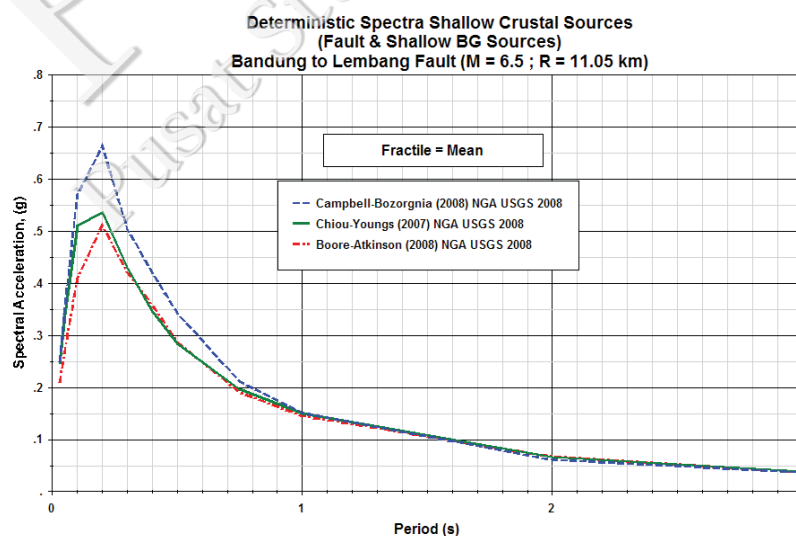
Gambar V-14. Grafik Respon Spektra untuk sumber gempa Shallow Crustal (Fault dan Shallow Background ) (Asrurifak, 2010)
